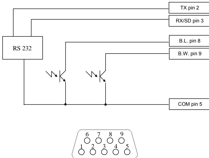
Sub D 9 Pin Buchsen (Computer Schnittstellen-Verbinder)
