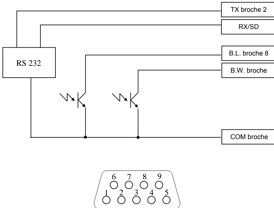
Sub D 9 broche femelle (connecteur interface ordinateur)
